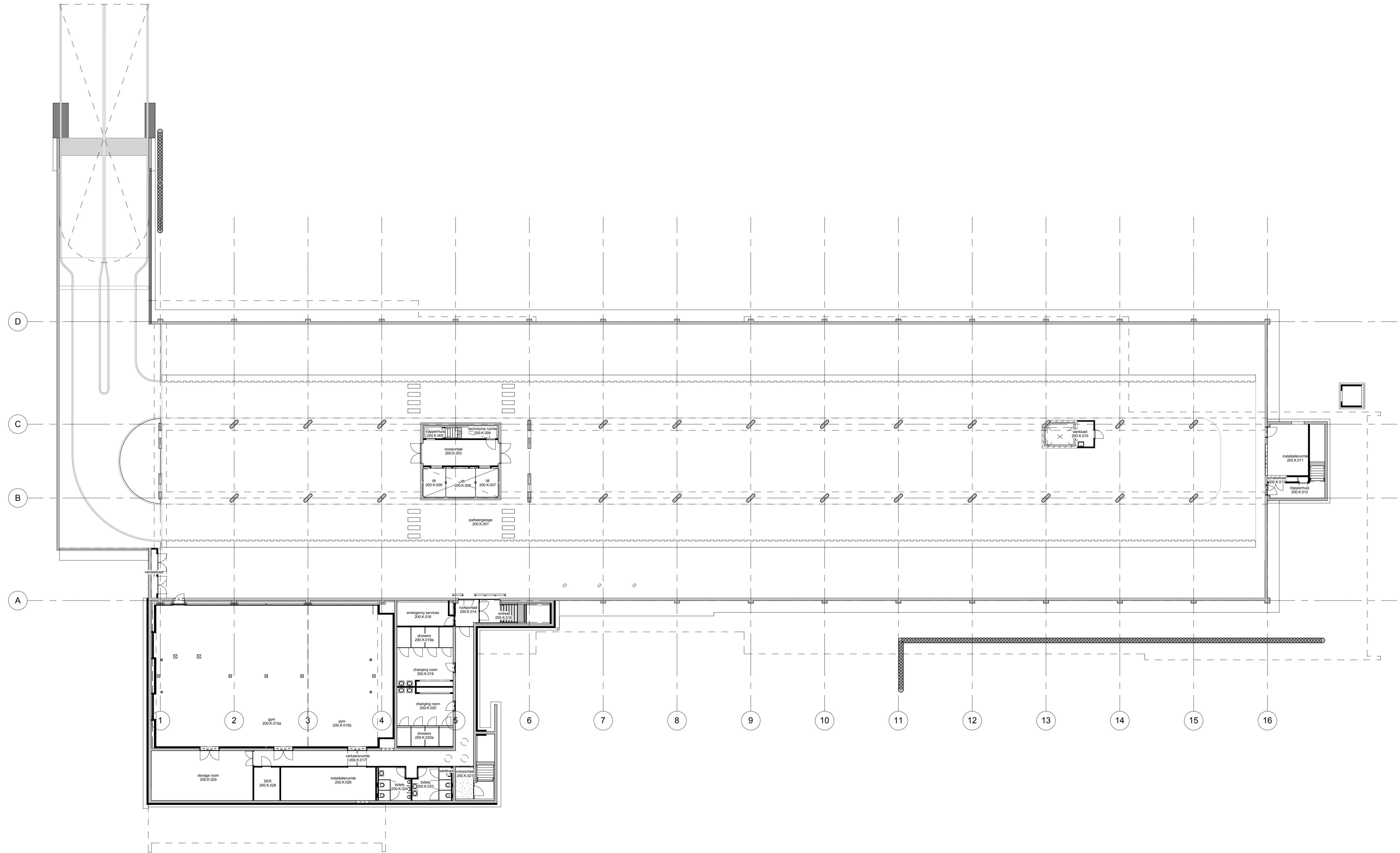
-1_Kelder schaal 1 : 200
